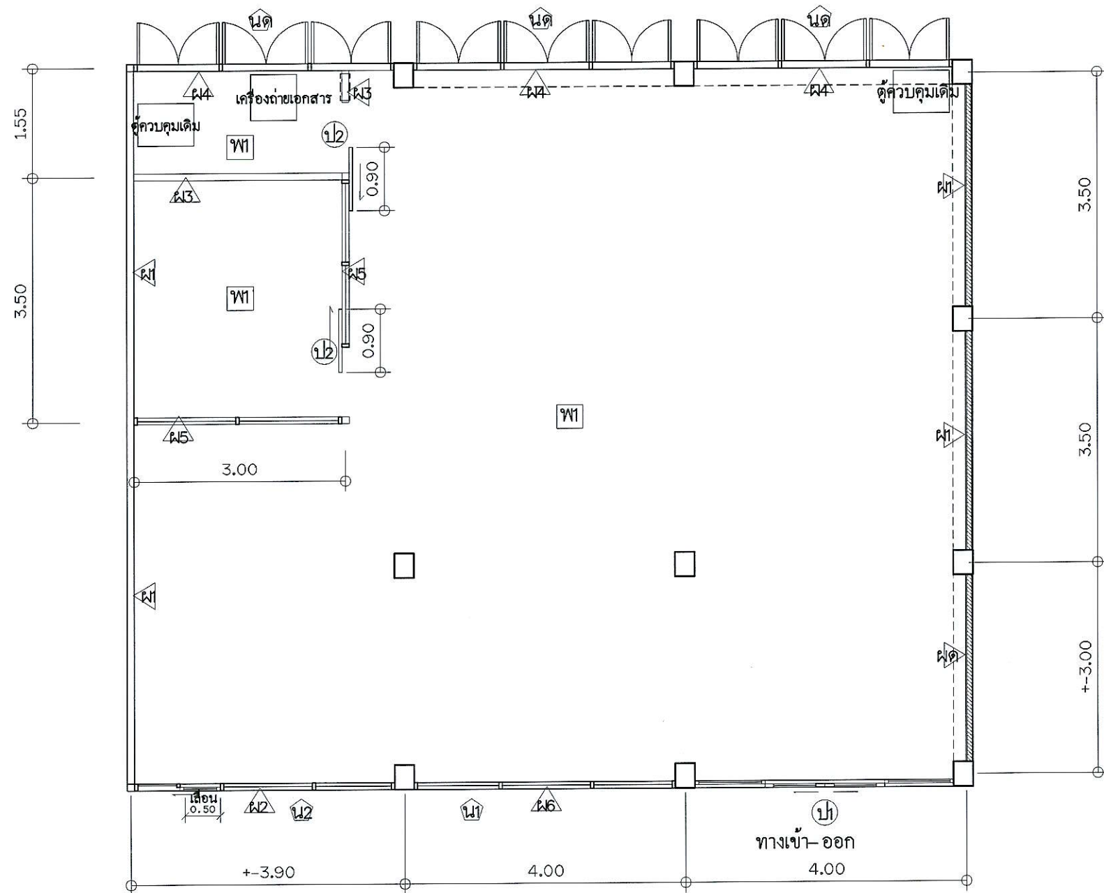
ผังพื้นที่ชั้นล่าง มาตราส่วน 1:75
