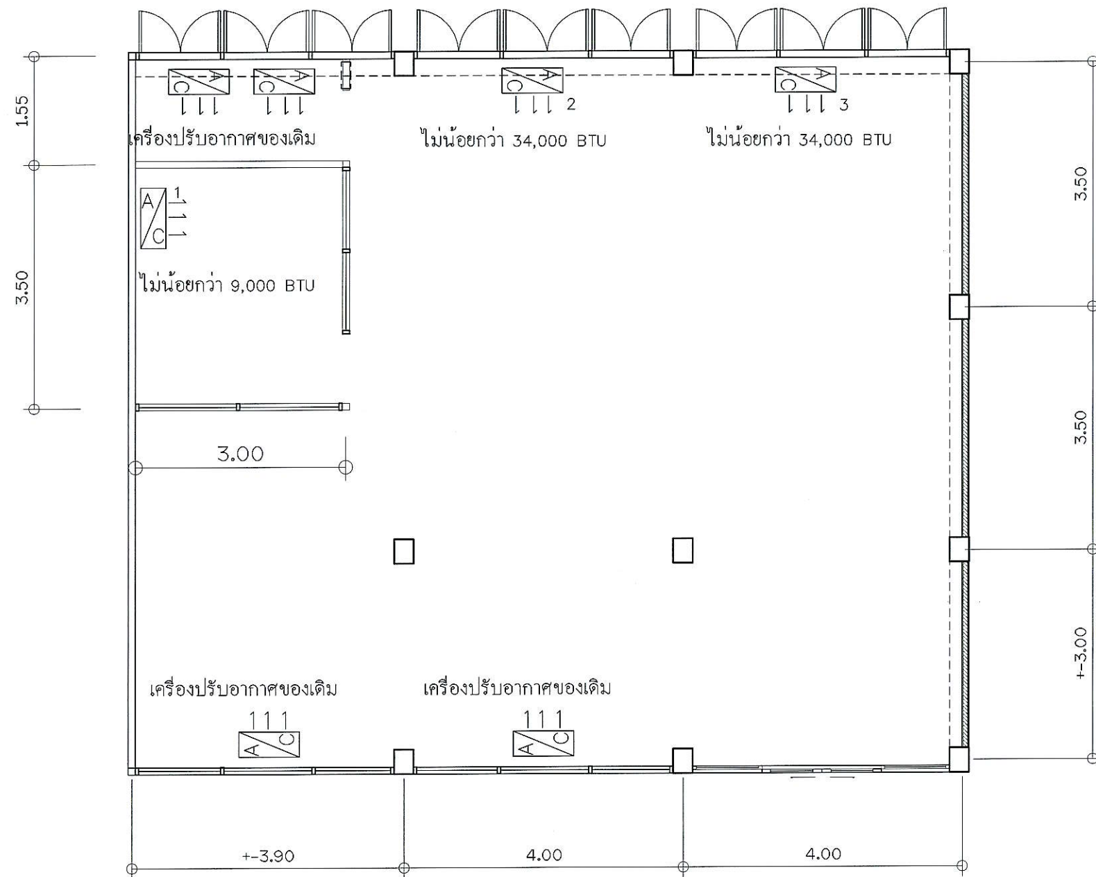
แปลนเครื่องปรับอากาศ มาตราส่วน 1:75
